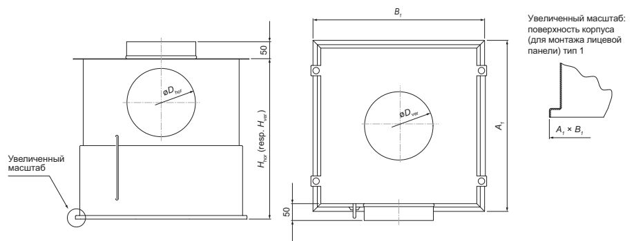
Рис. 3 Корпус CFC-G
