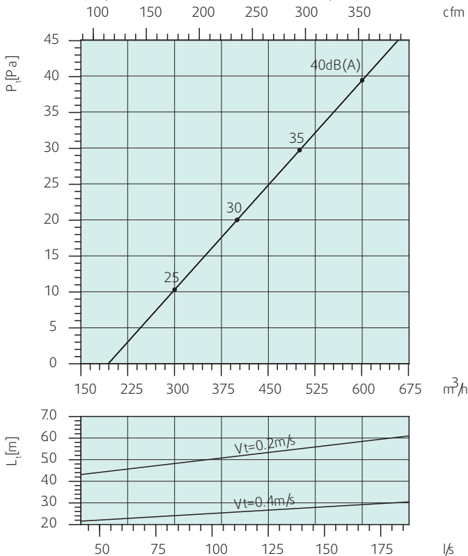
TSD - 315 Режим охлаждения (горизонтальная подача воздуха)
