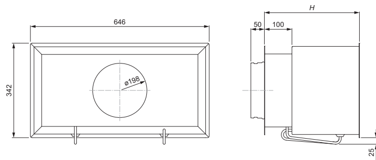
Рис. 5 Диффузор CFC-W, типоразмеры
