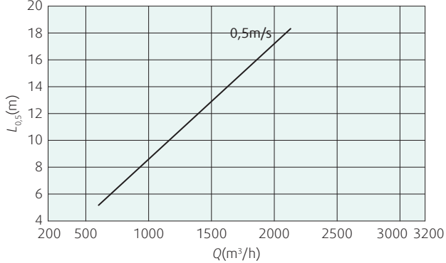
Диаграмма 3b: Дальность изотермической вертикальной струи 5-й позиции привода. Данные для конечной скорости 0,5м/с.
