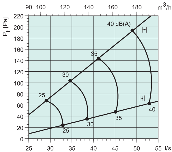
Sinus-A 160-S + THOR 125
