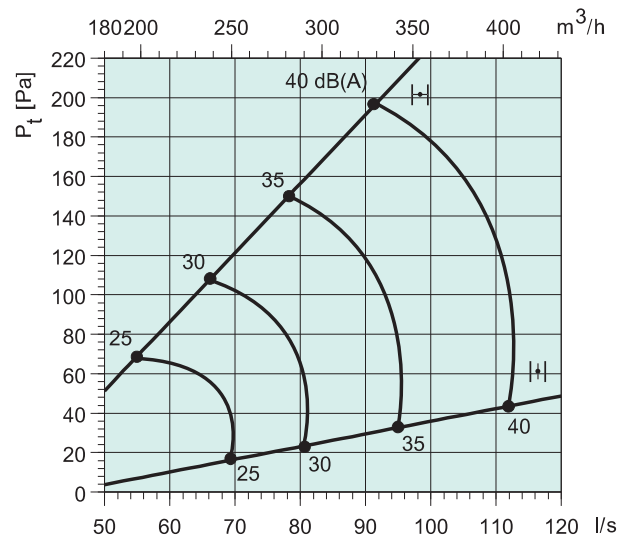
Sinus-A 250-L + THOR 200
