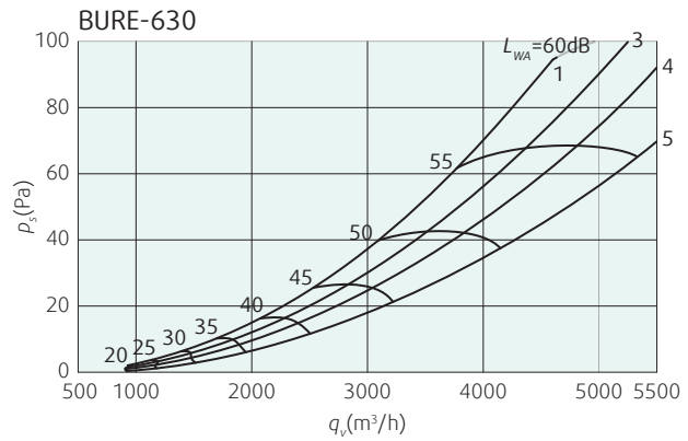
Диаграмма 5а: Падение давления и уровень звуковой мощности
