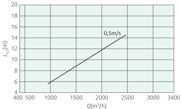
Диаграмма 4b: Дальность изотермической вертикальной струи 5-й позиции привода. Данные для конечной скорости 0,5м/с.
