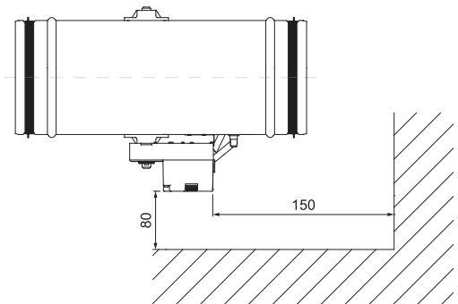
Установка Optima-R-BLC. Минимальное расстояние до стены
