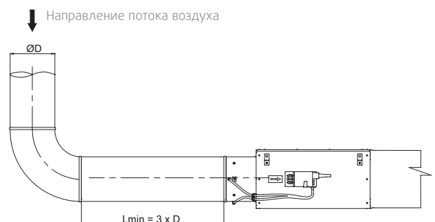
Установка Optima-RS-BLC. Минимальное расстояние до стены
