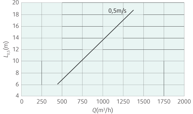
Диаграмма 2b: Дальностью изотермической вертикальной струи 5-й позиции привода. Данные для конечной скорости 0,5м/с.
