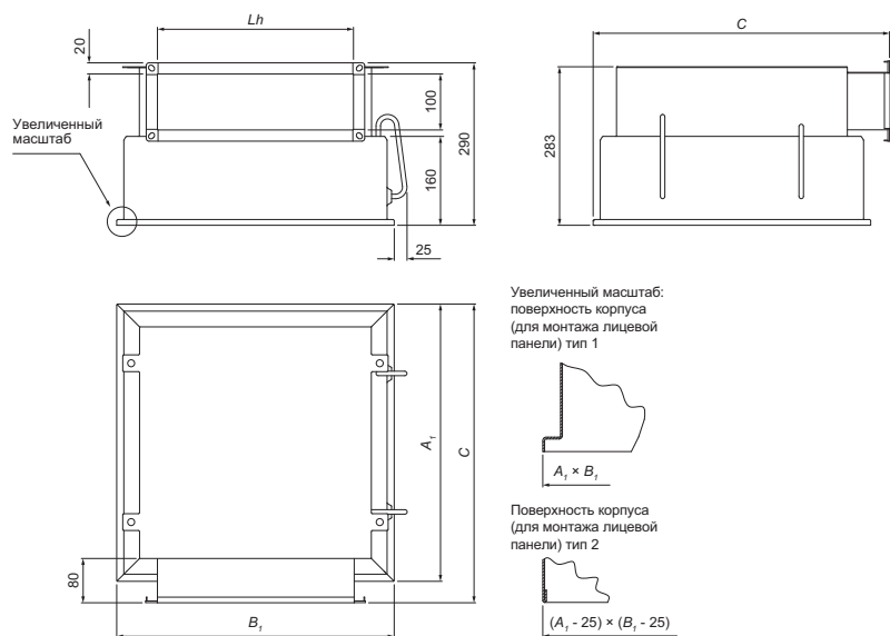
Рис. 4 Корпус CFC-R (прямоугольное подсоединение)
