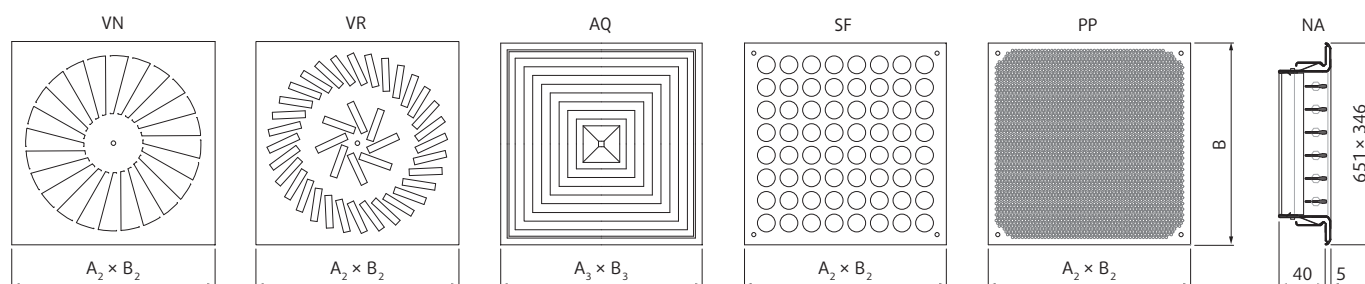
Таб. 10 Типоразмеры лицевых панелей CFC
