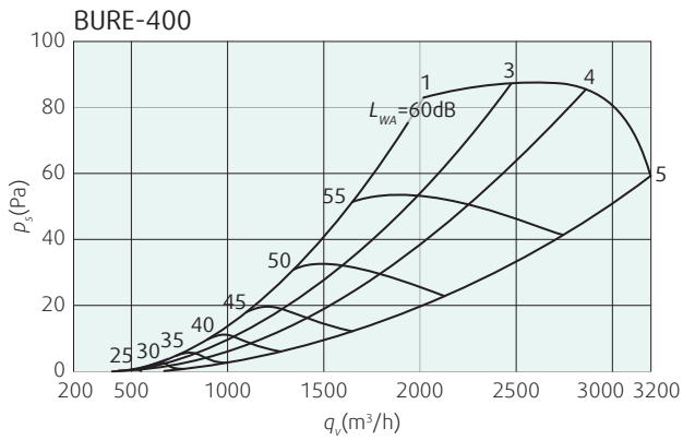
Диаграмма 3а: Падение давления и уровень звуковой мощности
