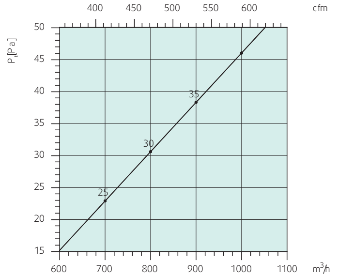
TSD-400 Режим отопления (вертикальная подача воздуха)
