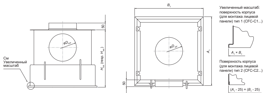
Рис. 1 Корпус CFC-C (Classic). H_{\text{гор}} - горизонтальное, H_{\text{вер}} - вертикальное присоединение.
