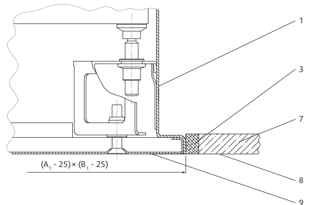
Рис. 8 Монтаж CFC, тип 1 в подвесной металлический потолок
