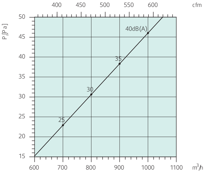
TSD - 400 Режим охлаждения (горизонтальная подача воздуха)
