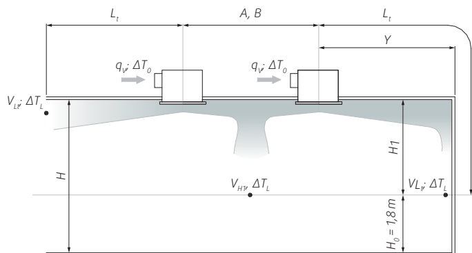
Распределение воздуха в помещении
