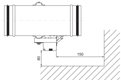
Установка Оптим-Р-ВЛС. Минимальное расстояние до стены
