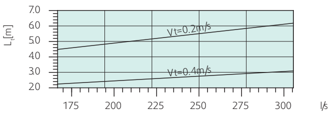
TSD - 630 Режим охлаждения (горизонтальная подача воздуха)
