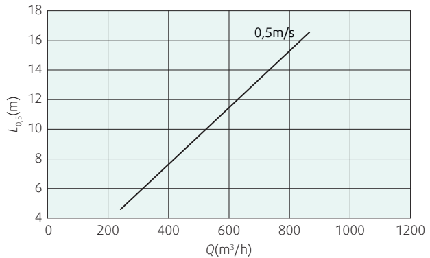
Диаграмма 1b: Дальностью изотермической вертикальной струи 5-й позиции привода. Данные для конечной скорости 0,5м/с.
