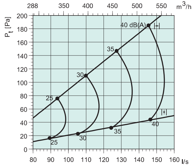
Sinus-A 315-L + THOR 250
