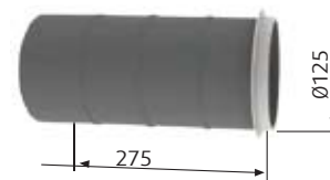
Проходной патрубок
