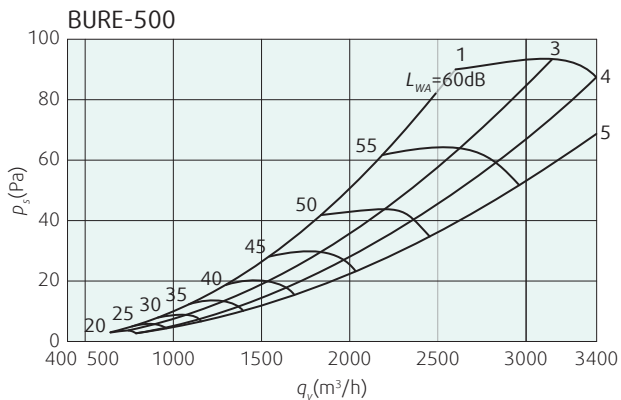
Диаграмма 4а: Падение давления и уровень звуковой мощности
