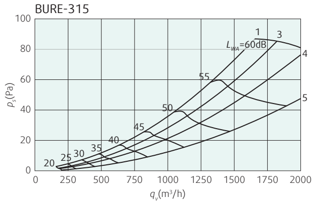
Диаграмма 2а: Падение давления и уровень звуковой мощности
