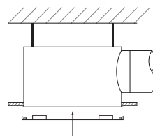
1. Установка западлицо в подвесные потолки
