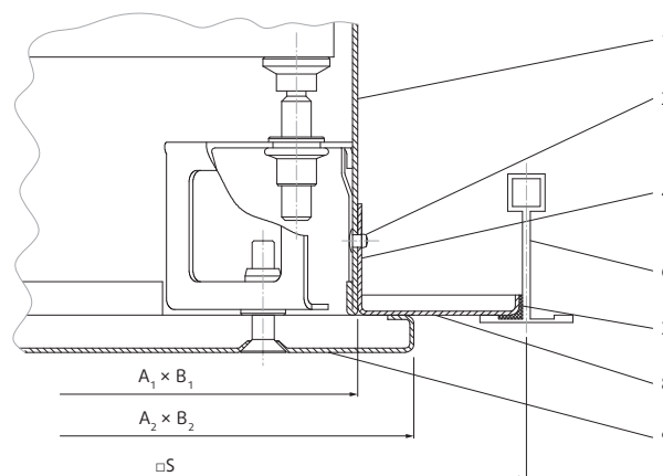
Рис. 10. Монтаж CFC, тип 1 в подвесной потолок T-bar
