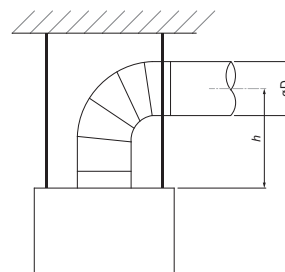
2. Свободно подвешанный к потолку диффузор h min > (3-5) D
