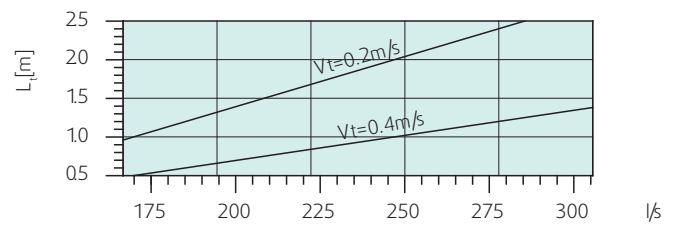
TSD-630 Режим отопления (вертикальная подача воздуха)
