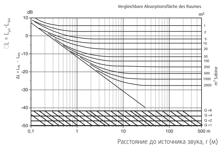
Рис. 3. Примерная оценка уровня звукового давления
