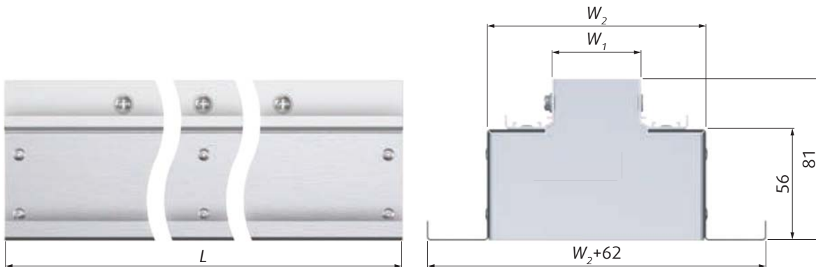
Fig. 1: Рис. BS-1-МВ, BS-2-МВ и BS-3-МВ
