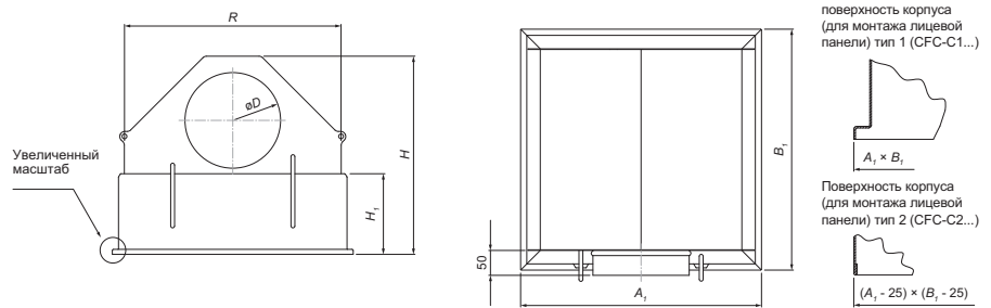
Рис. 2 Корпус CFC-B (Basic)
