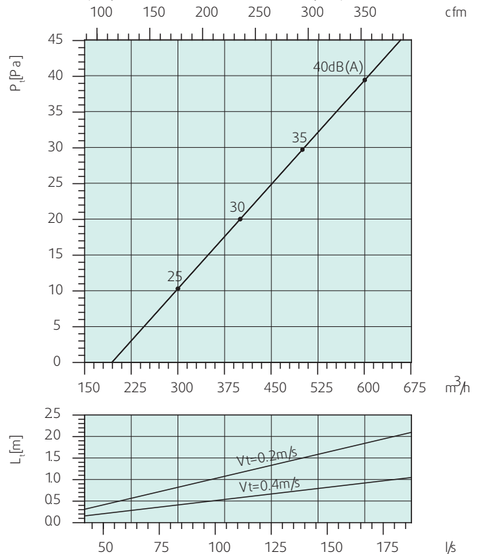
TSD-315 Режим отопления (вертикальная подача воздуха)
