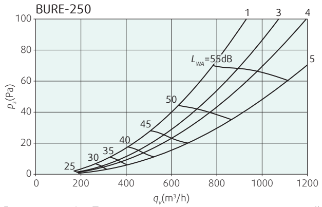
Диаграмма 1а: Падение давления и уровень звуковой мощности
