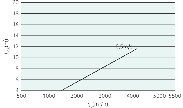
Диаграмма 5b: Дальность изотермической вертикальной струи 5-й позиции привода. Данные для конечной скорости 0,5м/с.
