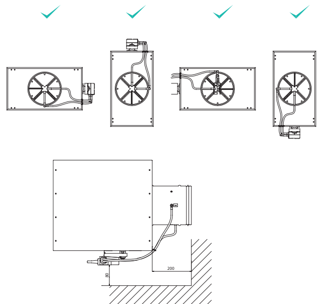
Установка Optima-RS-BLC. Минимальное расстояние до стены
